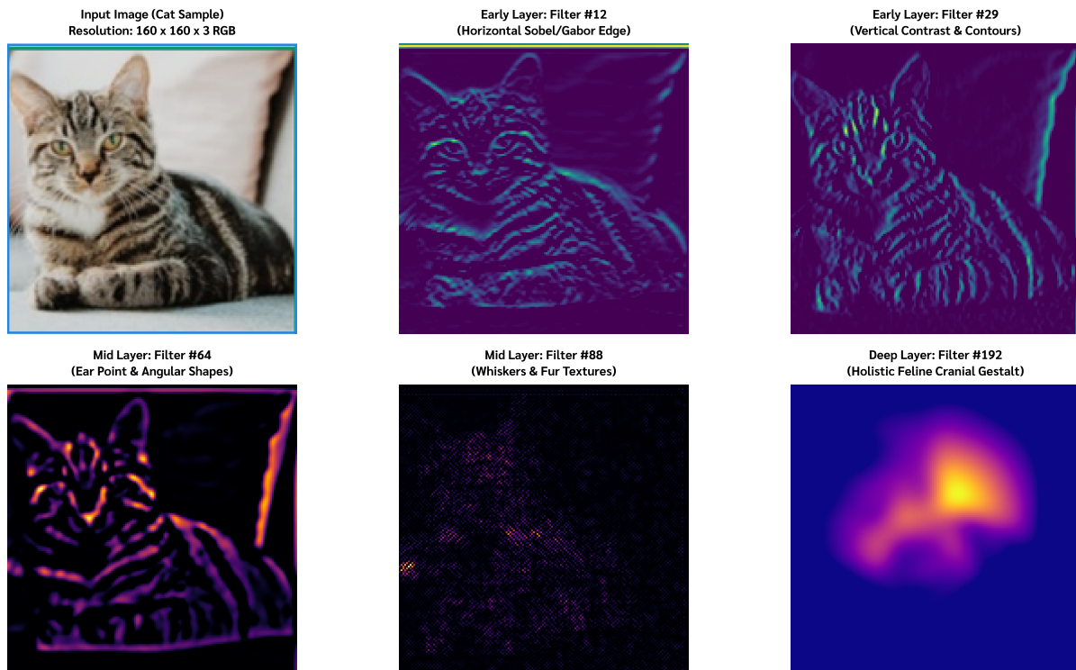
รูปที่ 5: การถอดรหัสฟีเจอร์ภายในโครงข่าย: วิวัฒนาการของ Receptive Field ตั้งแต่เลเยอร์ระดับต้น (block_1_expand_relu: ตรวจจับเส้นขอบ) ระดับกลาง (block_13_expand_relu: ตรวจจับลวดลายขนและมุม) จนถึงระดับลึก (out_relu: ตรวจจับอวัยวะสำคัญบนใบหน้า)
